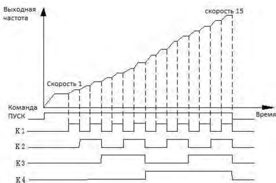
Рисунок F 4-1 Работа на многоступенчатой скорости
