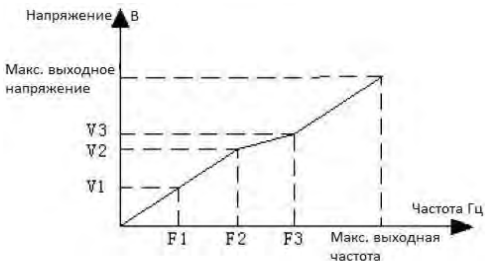
Рисунок F3-3 Настраиваемая пользователем кривая V / F
