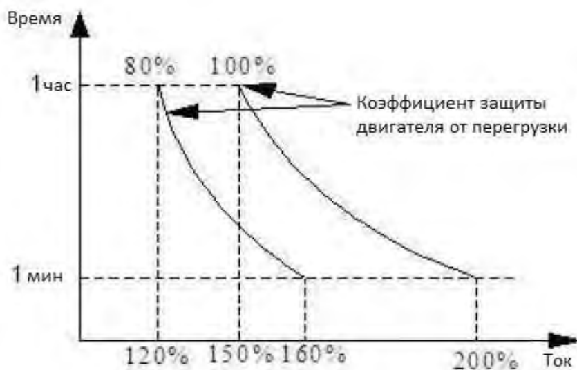
Рисунок F9-2 Установка коэффициента защиты двигателя от перегрузки Коэффициент рассчитывается по формуле ниже:
