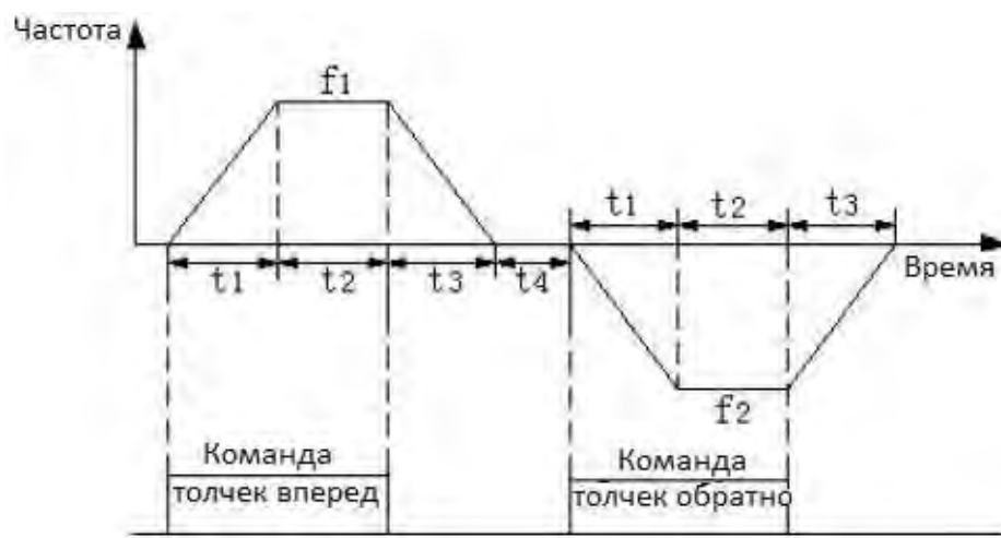
Рисунок F8-1 Толчковый режим
