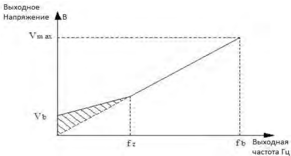
Рисунок F3-2 Повышение крутящего момента
