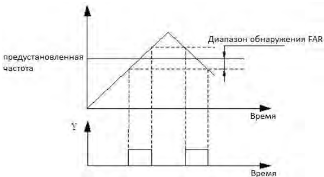
Рисунок F8-4 Достижение частоты
